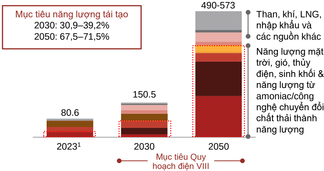
Năng lực điện đã lắp đặt của Việt Nam trong Quy hoạch điện VIII (GW)
